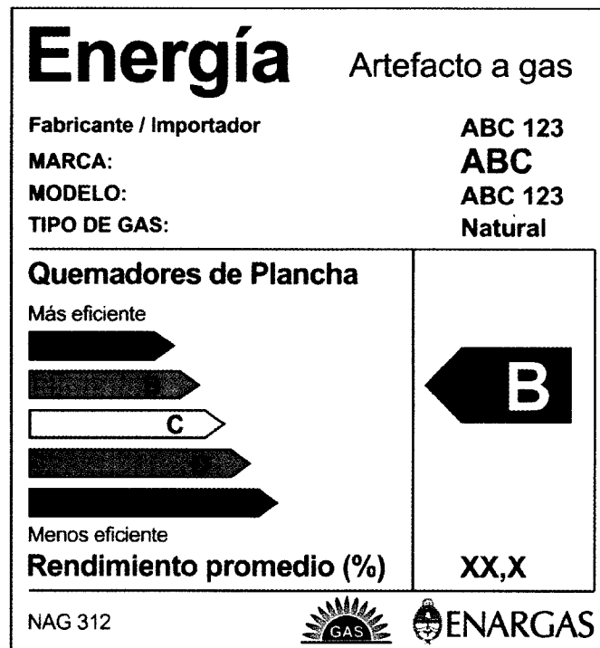
Figura E.2 - Etiqueta para aparatos de cocción a gas que poseen sólo quemadores de plancha
