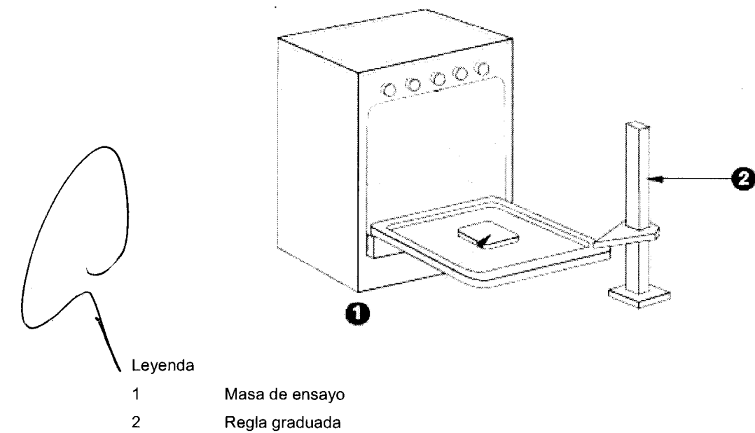
Figura 5 - Estabilidad de los accesorios del horno y del gratinador y resistencia de la puerta del horno (apartados 5.2.2.1, 5.2.2.2 y 5.2.2.3)
