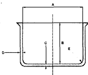
Figura C.1 - Recipientes necesarios para el ensayo de los quemadores de gas
