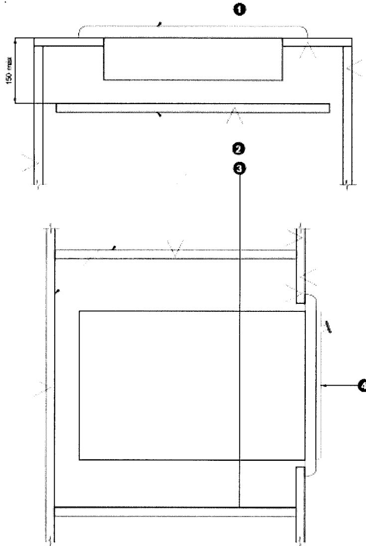
Figura 12 - Ejemplo de módulo de encastramiento para los artefactos de Clase 3 (apartados 5.1.2.2.3, 5.1.2.2.4.2.3 y 5.3.1.6.1.3)
