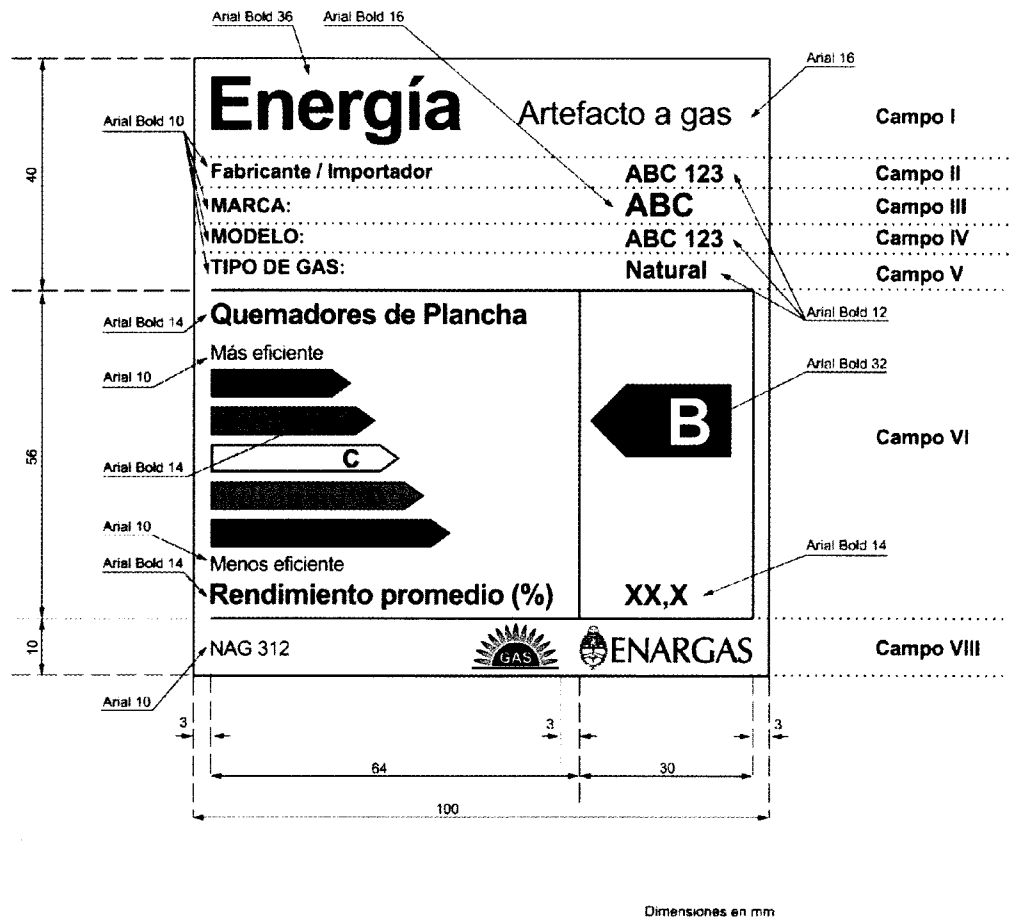
Figura E.5 - Diseño de la etiqueta para aparatos de cocción a gas que poseen quemadores de plancha y horno
