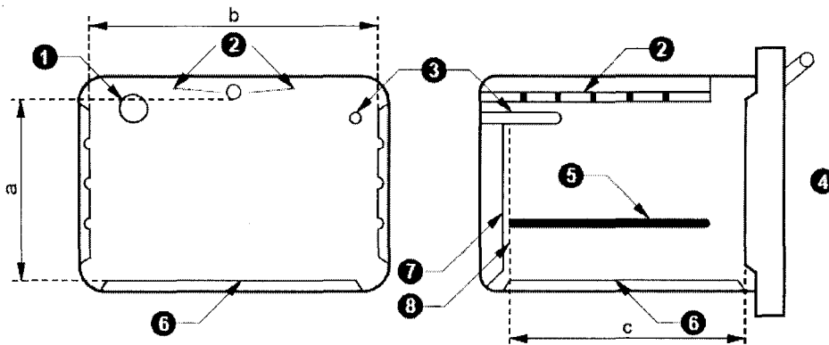
Figura 1 - Volumen útil del horno (apartado 1.4.3.37)
