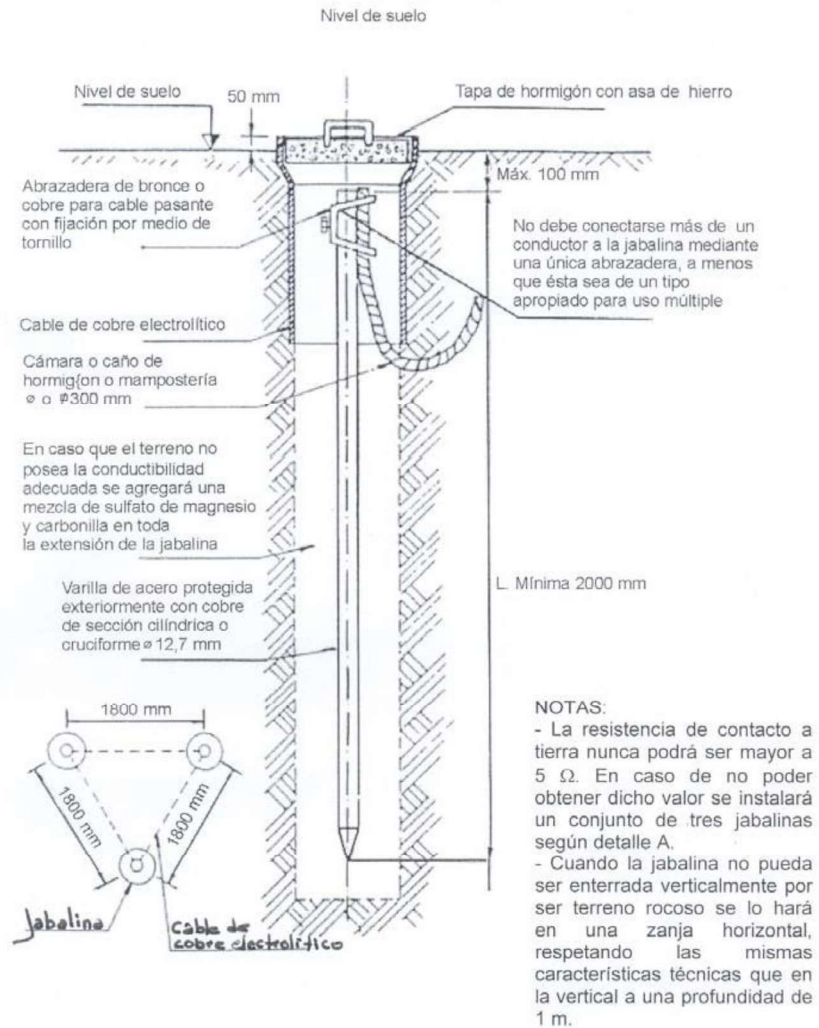
DETALLE A
